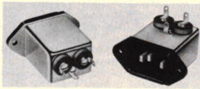
Afb. 2. Deze door Corcom uitgebrachte 50 Hz netfilters bevatten twee L-secties en condensatoren tussen beide fasen. Ze zijn goedgekeurd volgens VDE en IEC.
